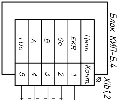
Х1.1 2РМ18КПНТГ1В1 (розетка на кабель)
