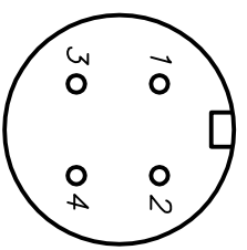
Розетка 2PМ14КПНЦГ1В1
