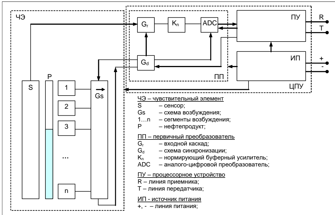
Рисунок 3: блок-схема уровнемера
